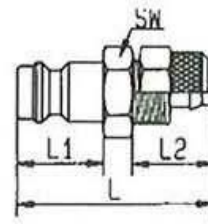
Nippel für Schlauch
