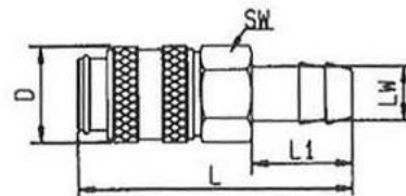
Schlauchtülle
